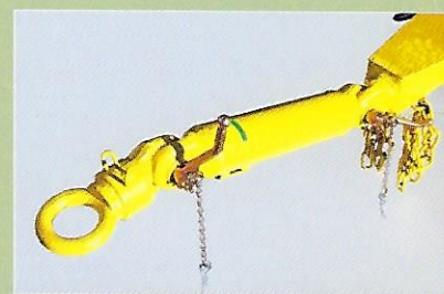
■ Timon double articulation avec anneau
